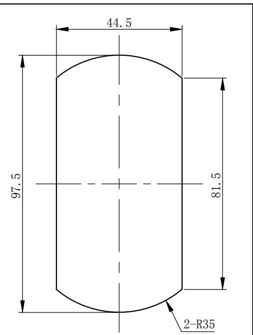
パネル穴明け寸法
