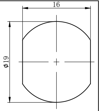
パネル穴明け寸法
