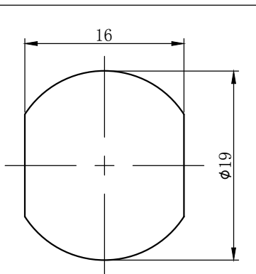
パネル穴明け寸法
